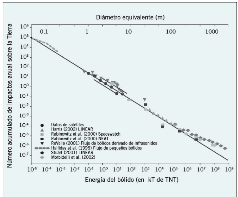
Fig. 5. Gráfica del flujo de cuerpos que chocan contra la Tierra en la actualidad. Se basa en las estadísticas obtenidas por programas de seguimiento de NEOs, detección de superbólididos mediante satélites artificiales o infrasonidos y para objetos por debajo de 1 metro las redes de seguimiento de bólidos. Adaptada de Trigo-Rodríguez (2012) en base a un diagrama de Peter Brown (Univ. Western Ontario).
