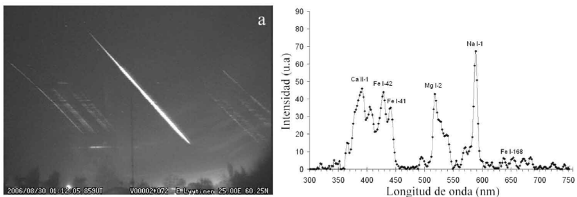
Figura 2. Izquierda. Espectro del bólido Lahti (FN 300806) registrado en Helsinki. Derecha. La descomposición en líneas espectrales del bólido ha permitido determinar la composición química del meteorite. Fuente: E. Lyytinen / J. M. Trigo / CSIC.
