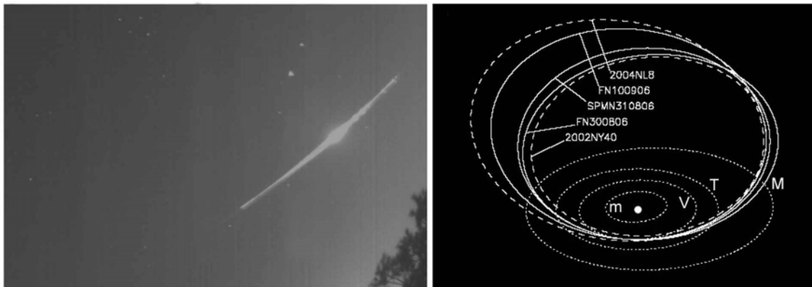
Figura 1. Izquierda. El bólido Cortes de la Frontera, producido por una roca de 10 kilos procedente del asteroide 2002NY40. Imagen tomada desde la estación de La Mayora del Instituto de Astrofísica de Andalucía (CSIC). Derecha. Órbitas de los asteroides 2002NY40 y 2004NL8 comparadas con las de los tres meteoroides del estudio. Fuente: J. M. Trigo / A. Castro-Tirado / D. C. Jones / CSIC.
